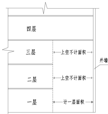
图 6.2.3 跨层部位、上空部位面积计算图示
