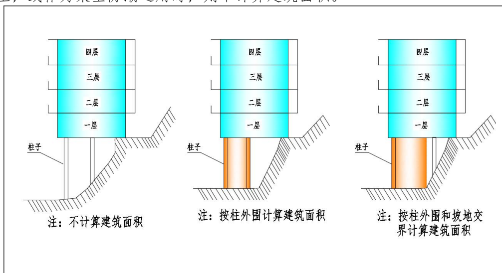
图 6.2.5.1 吊脚楼面积计算图示 1
