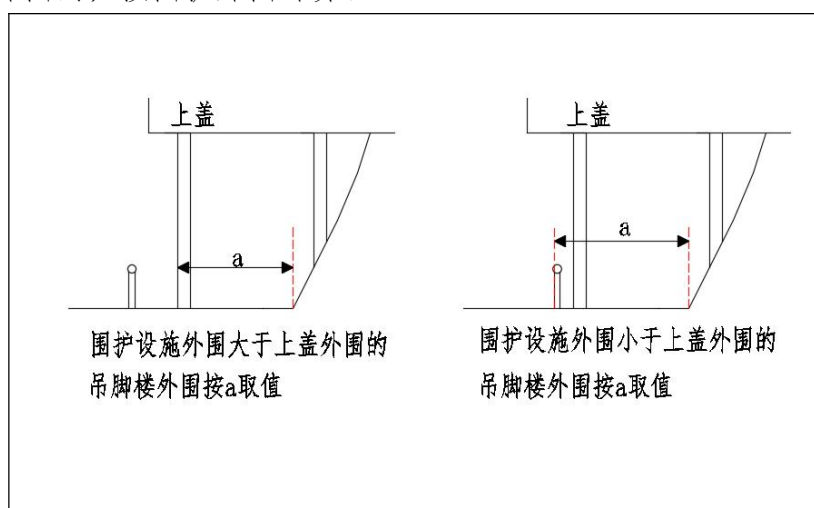
图 6.2.5.2 吊脚楼面积计算图示 2
